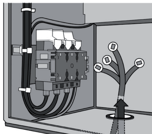
Apertura nel fondo del quadro elettrico e morsettiera per la linea d'alimentazione elettrica
