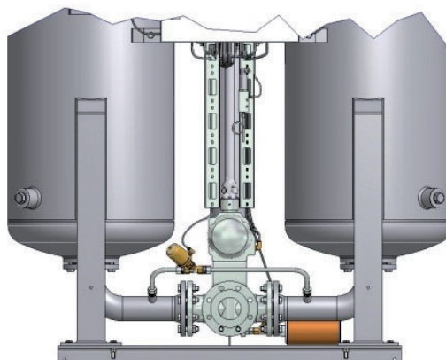
Ingresso dell'aria compressa dell'essiccatore
